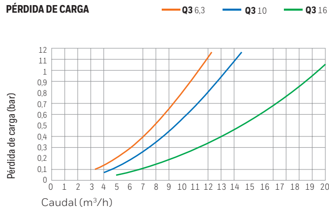
PÉRDIDA DE CARGA
